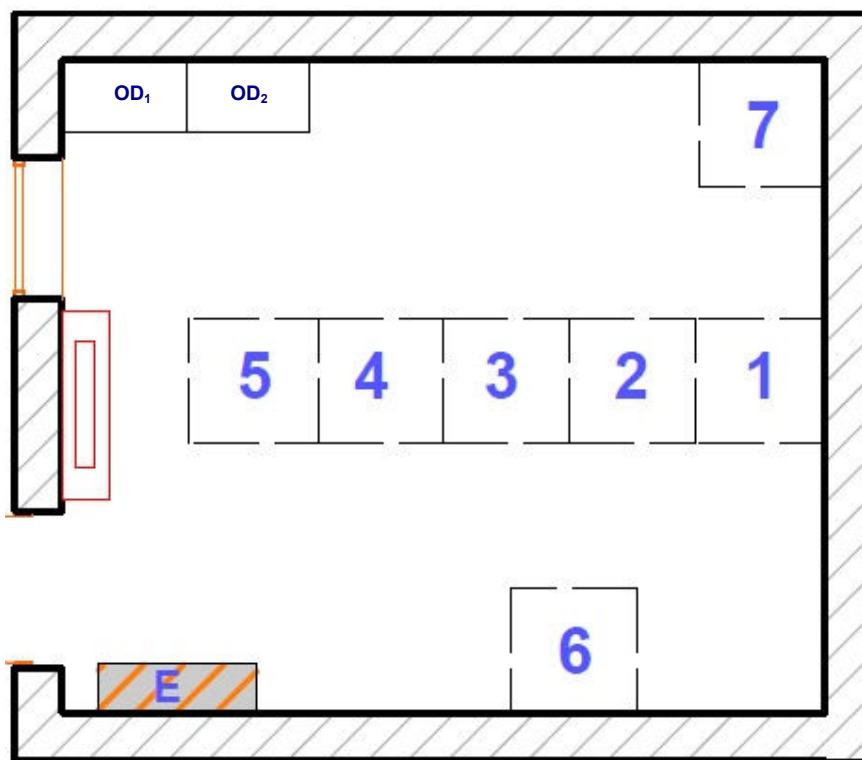
Slika 6: Shematski prikaz lokacije Senuše z mesti za postavitev komunikacijskih omar
